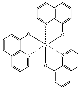
Alq 3
